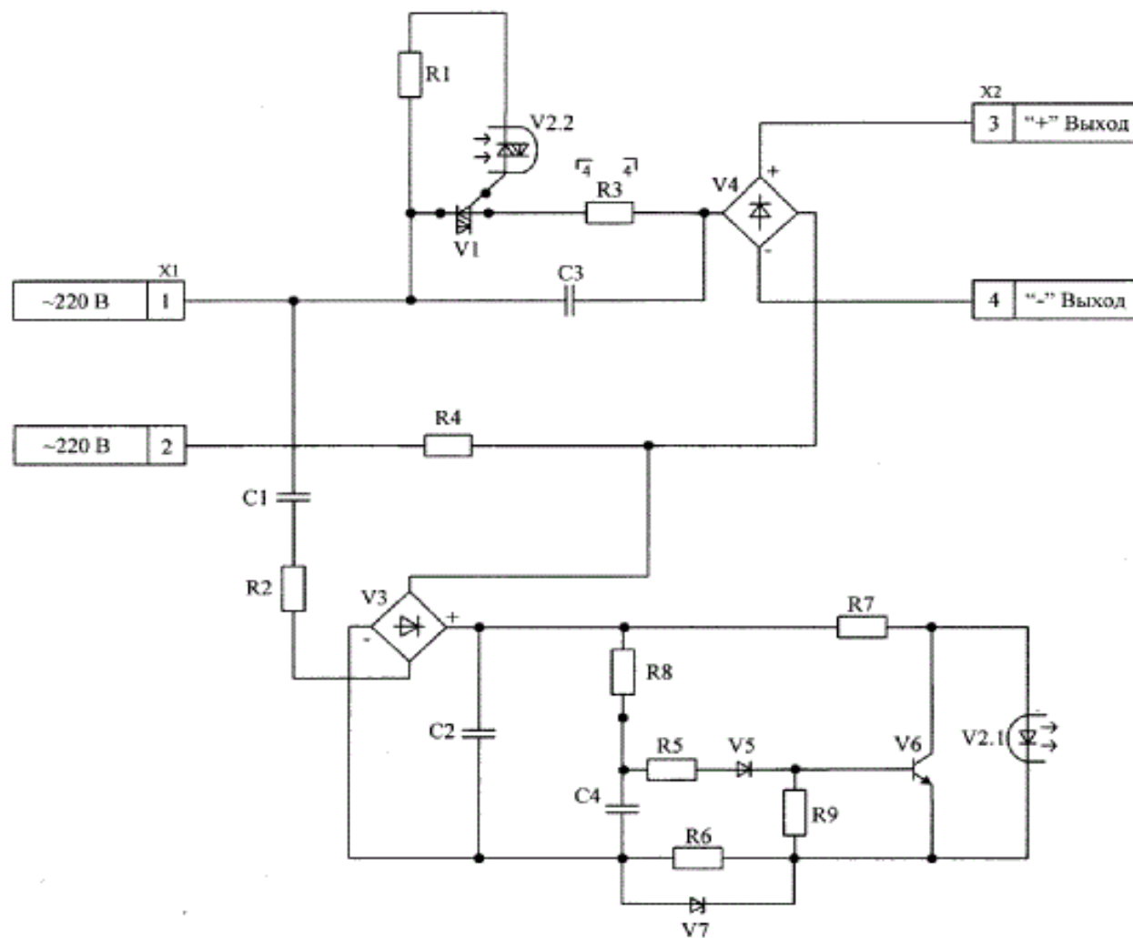
Схема электрическая принципиальная ФУТ-1М
